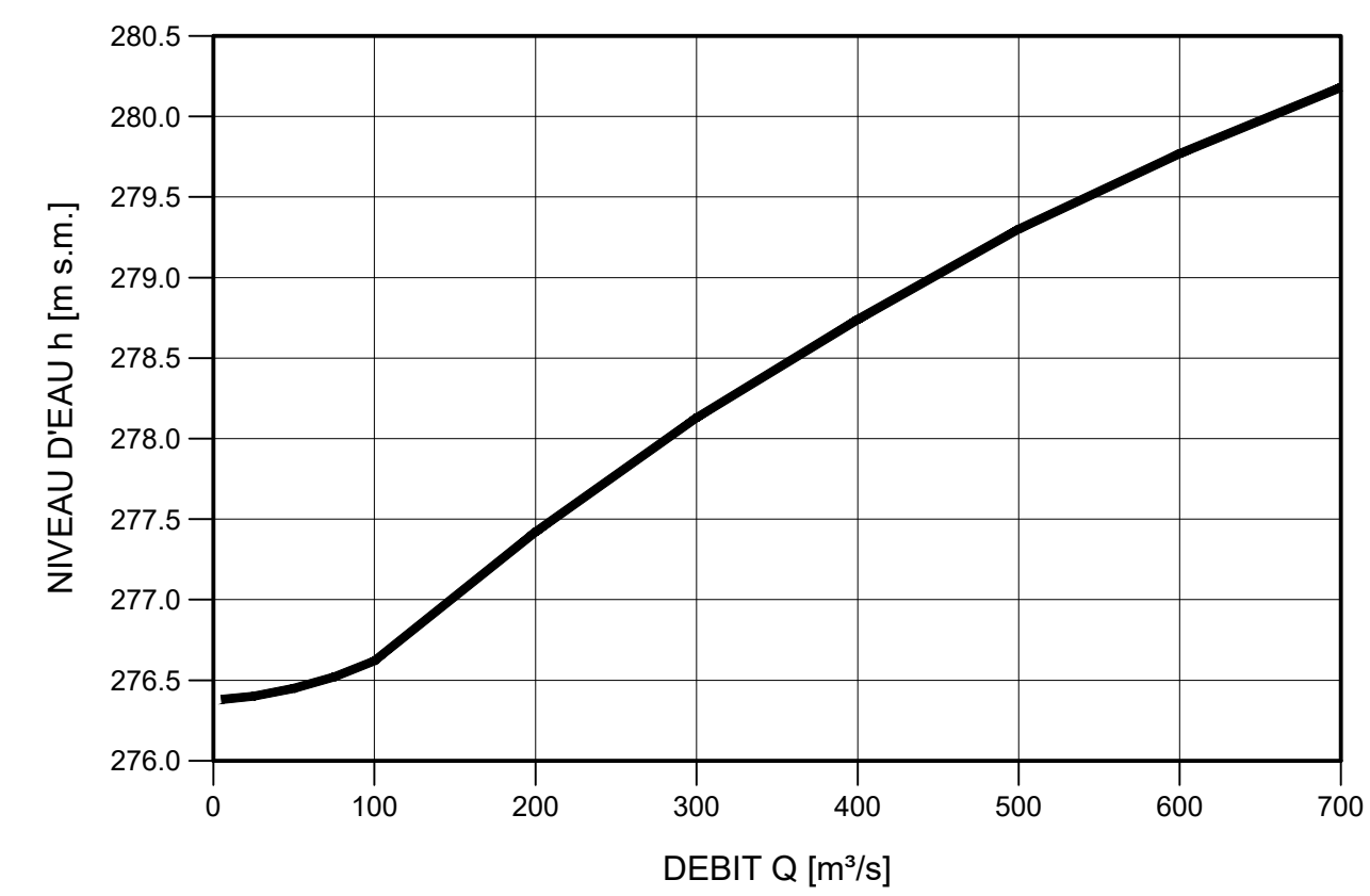
EVOLUTION DU NIVEAU DE LA SURE h DANS LA SECTION DE TARAGE EN FONCTION DU DEBIT Q
