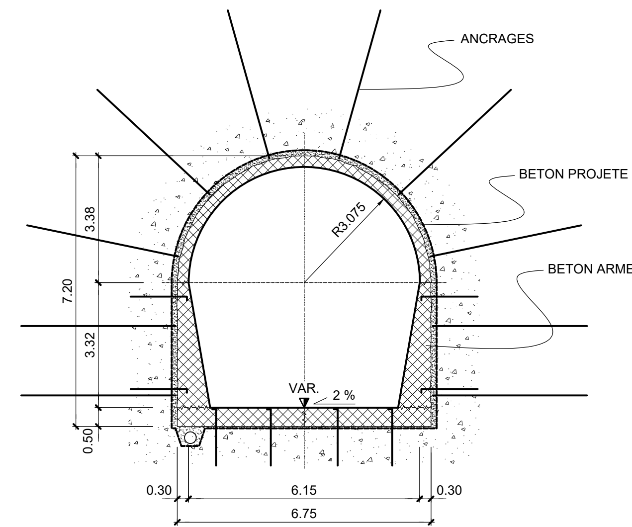
COUPE B-B
