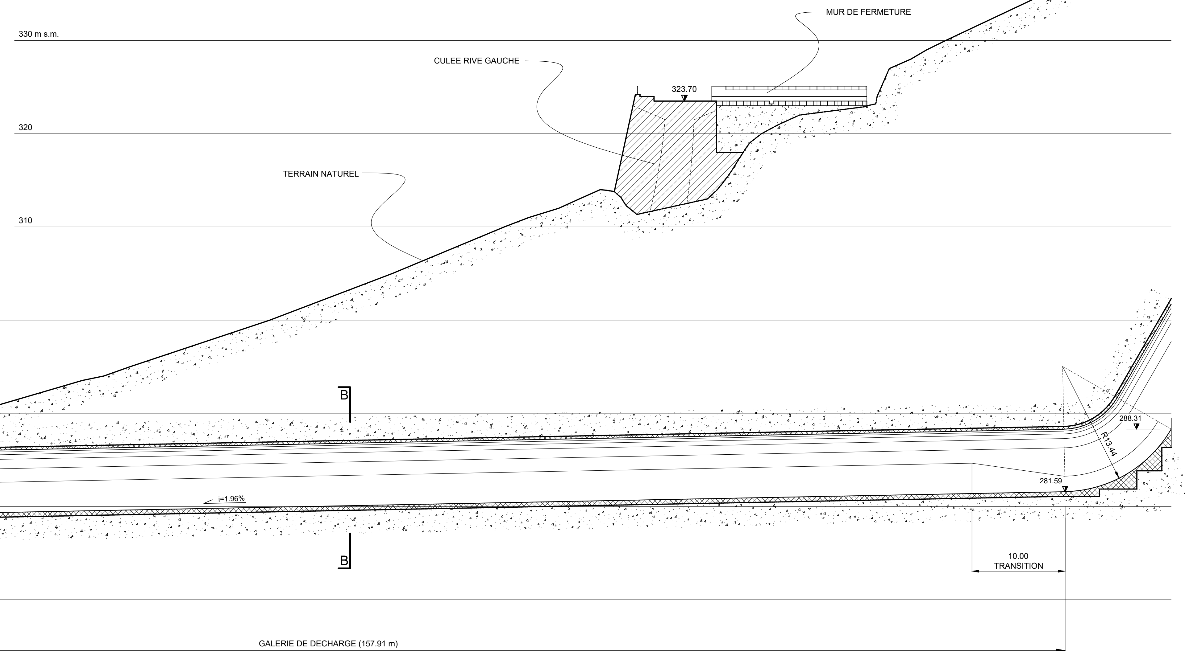
GALERIE DE DECHARGE - PROFIL LONGITUDINAL
